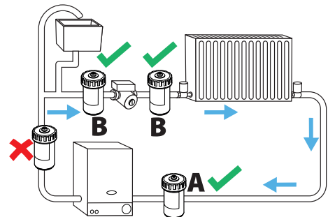
开放式通风系统
