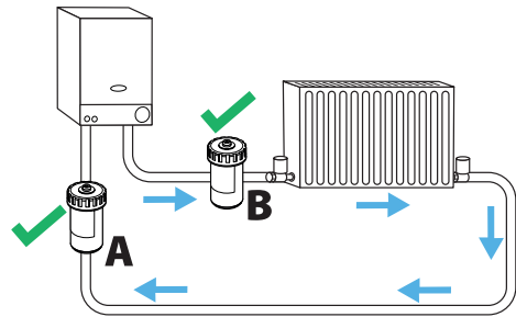
复式/密闭系统
